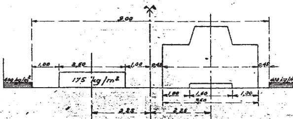
Chaussée de 9,00m
