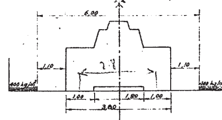
Chaussée de 6,00m
