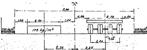
Chaussée de 9,00m
