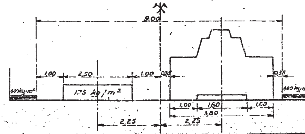
Chaussée de 9,00m
