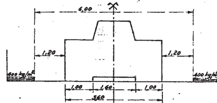
Chaussée de 6,00m
