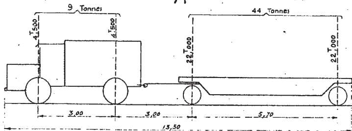
Véhicule type de 2 ème classe
