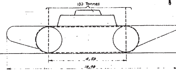
Chaussée de 6,00m
