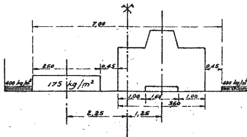
Chaussée de 7,00m
